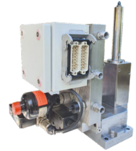
Injektionsmodul mit Ventilbaugruppe
